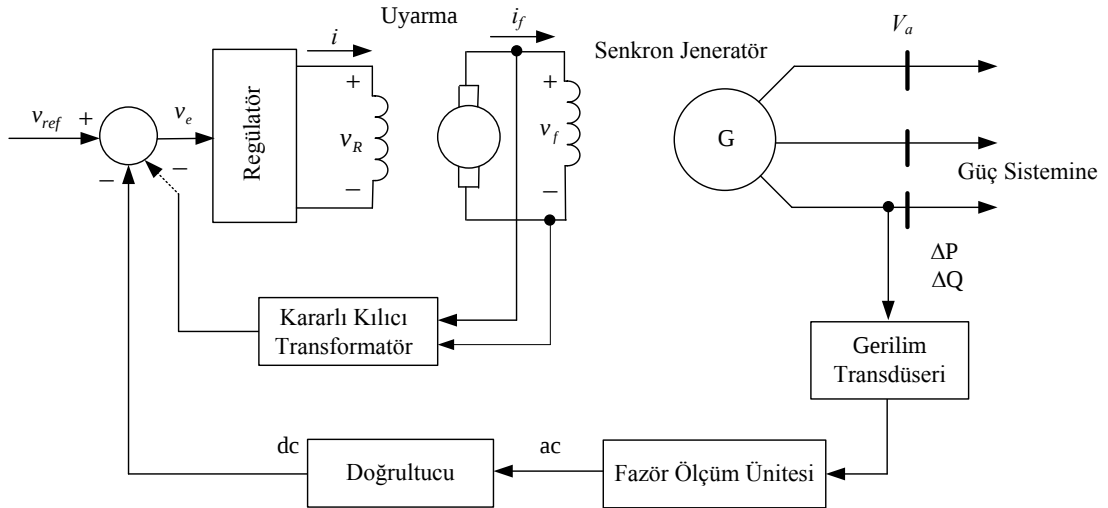
Şekil 1.1: Senkron jeneratör uyarma kontrol sisteminin diyagramı
